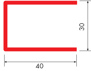
6040-7060 Kapı / Door
